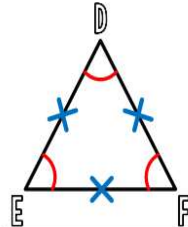
le triangle équilatéral
