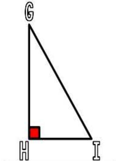
le triangle rectangle
