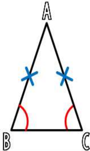
le triangle isocèle
