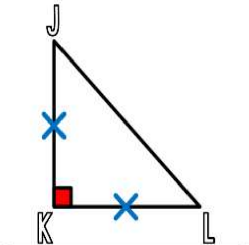
le triangle isocèle rectangle
